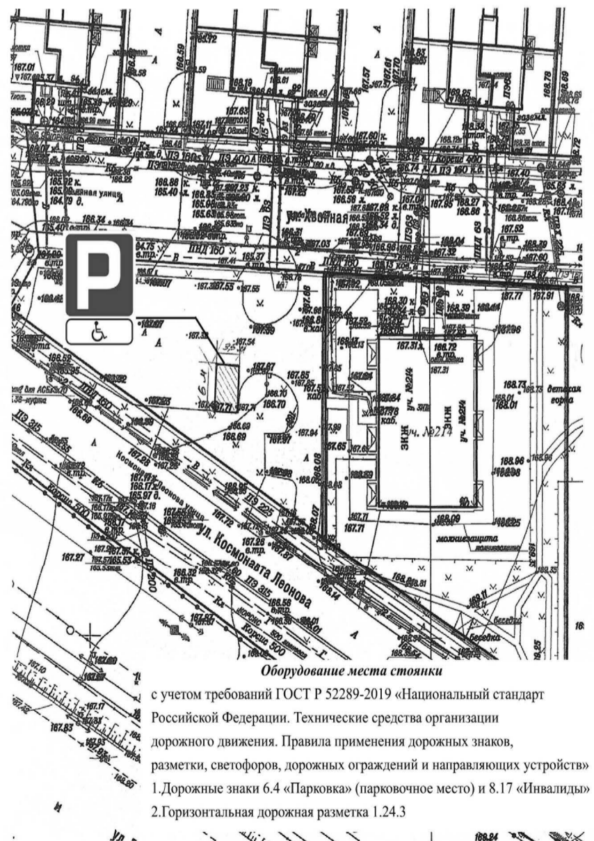
Схема размещения автомобиля, перевозящего инвалида, выполненная на топографической съемке в масштабе 1:500, вблизи дома 60 по ул. Космонавта Леонова г. Обнинска
